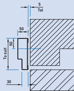
Optional Frame Profile
