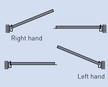
Double blade inward opening
