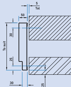
Optional Frame Profile
